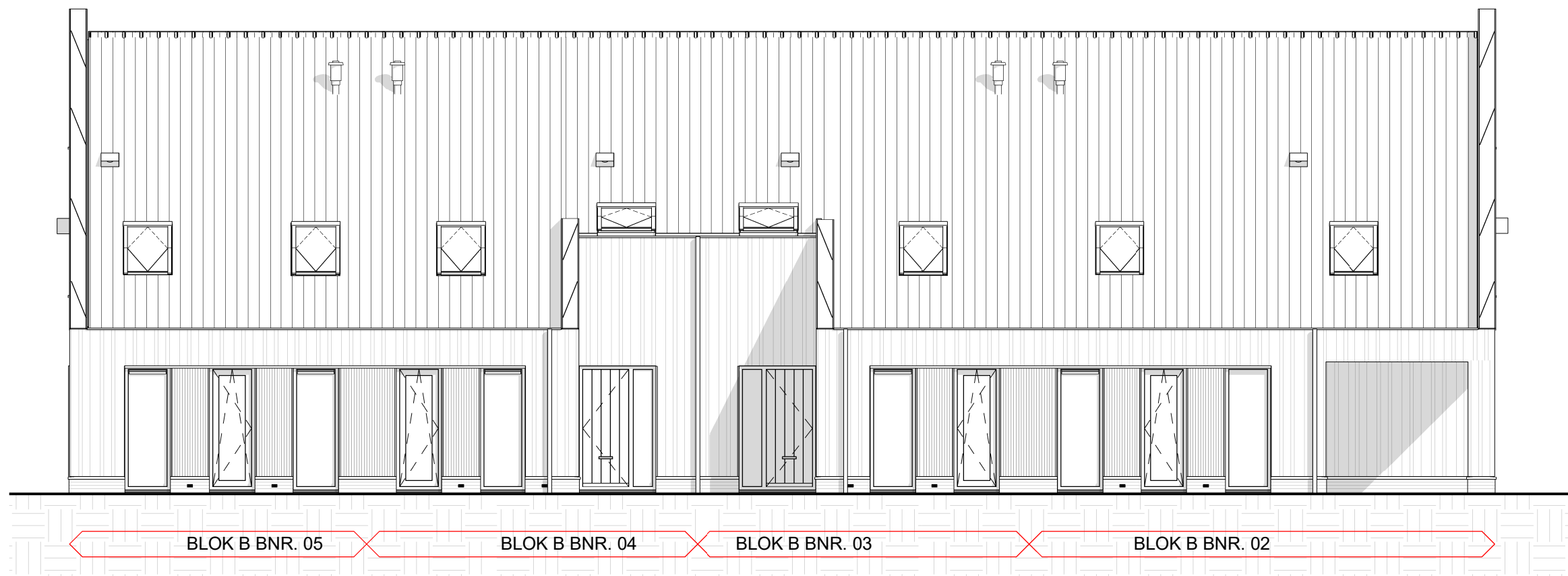
voorgevel
