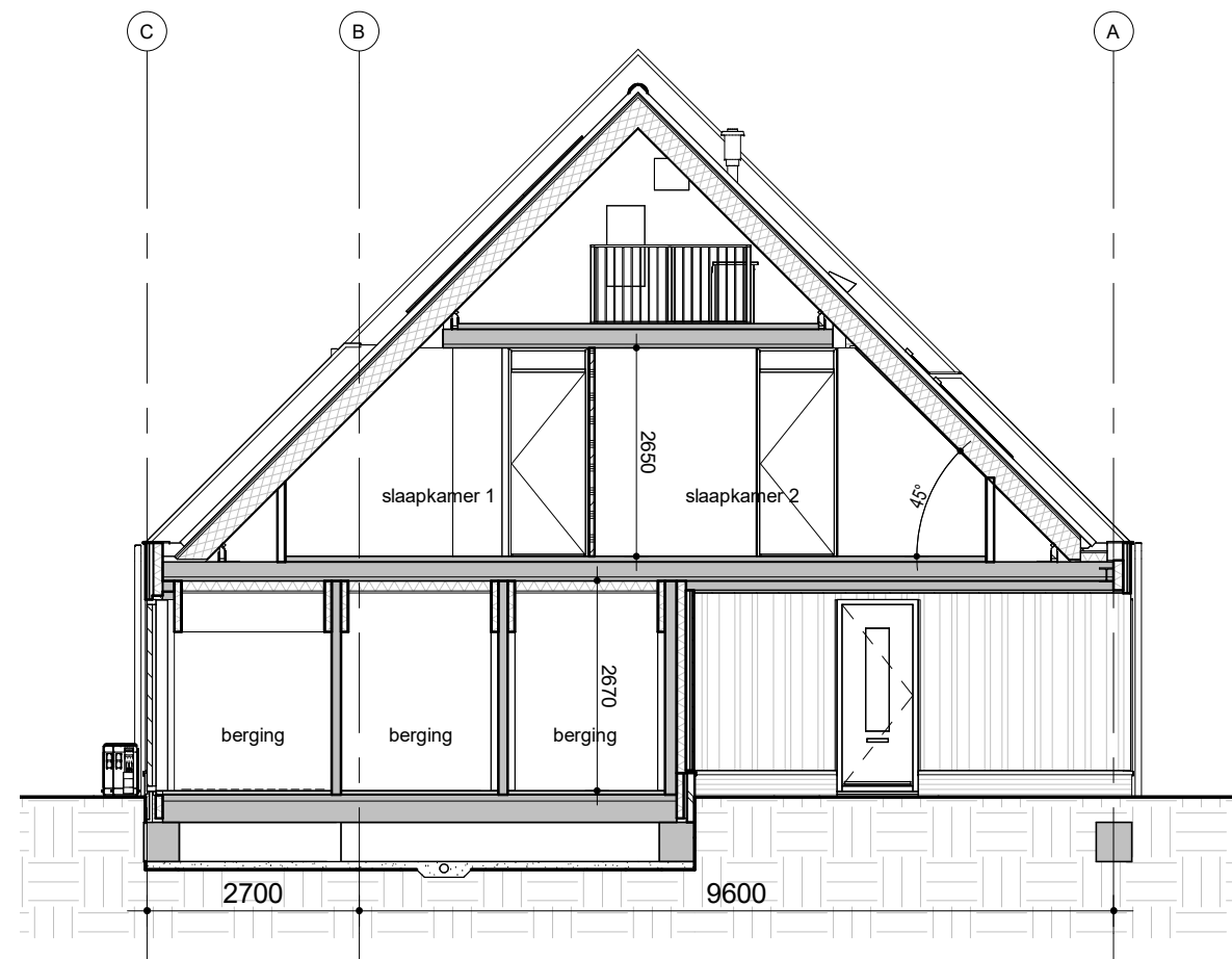
doorsnede C
