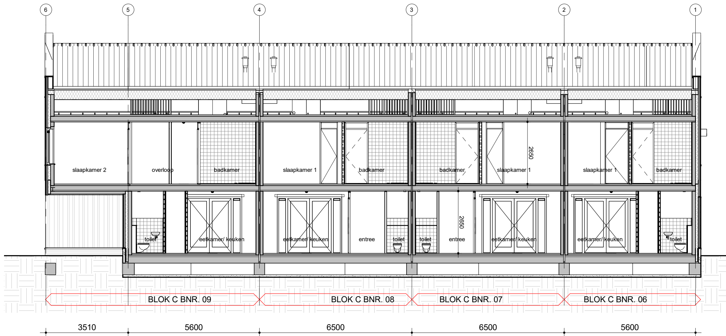
Doorsnede D
