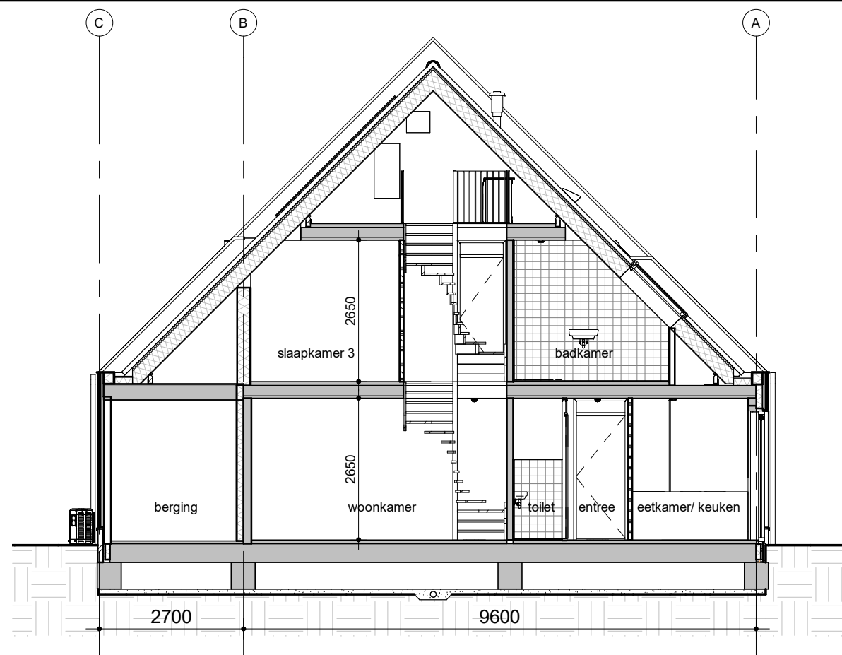
Doorsnede A
