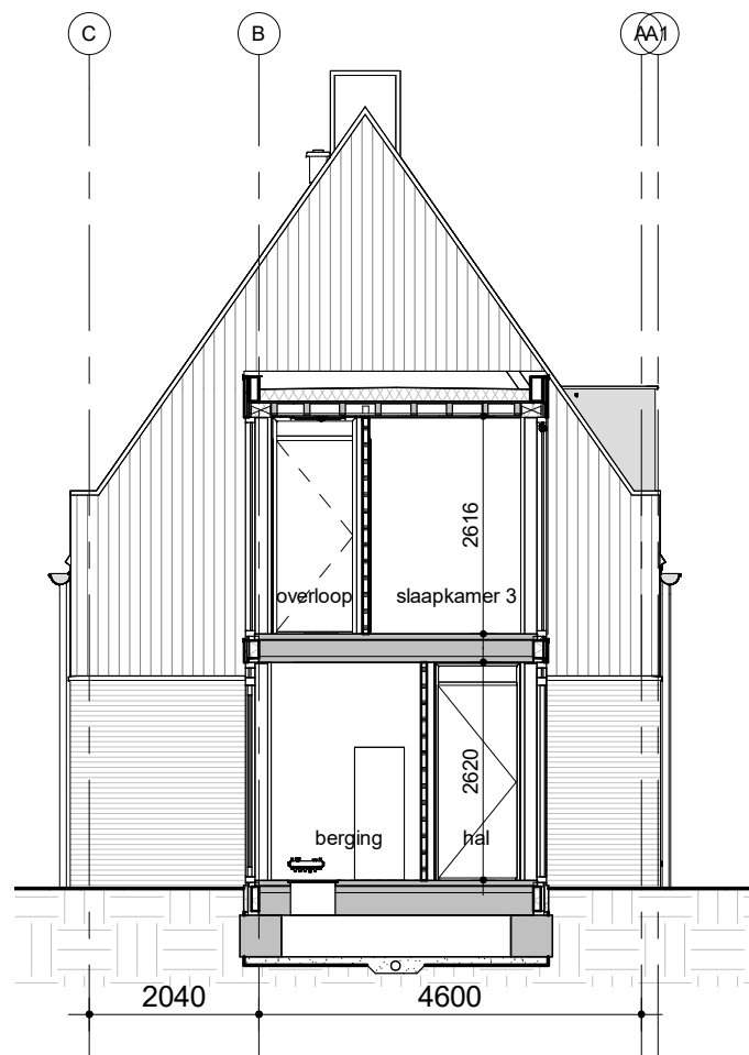
Doorsnede A
