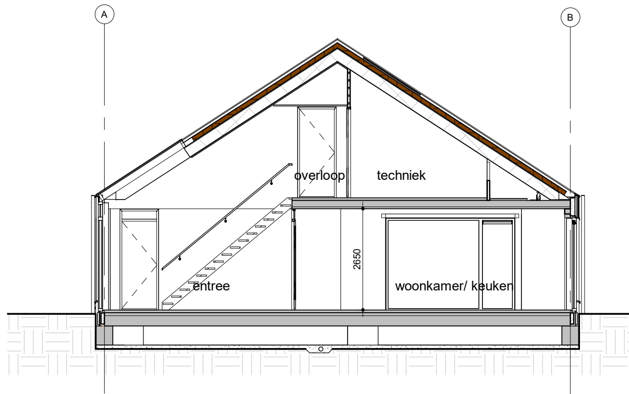
Doorsnede A
