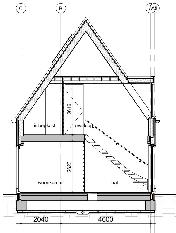
Doorsnede B
