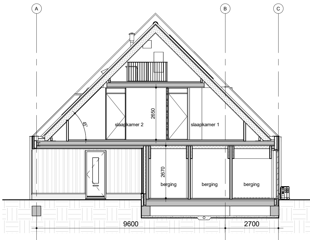
Doorsnede C
