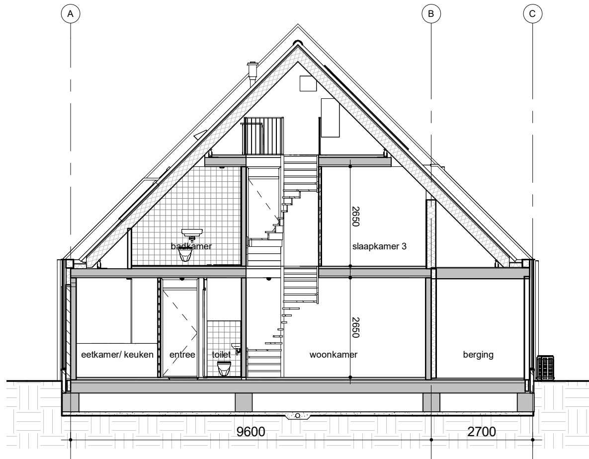
Doorsnede A
