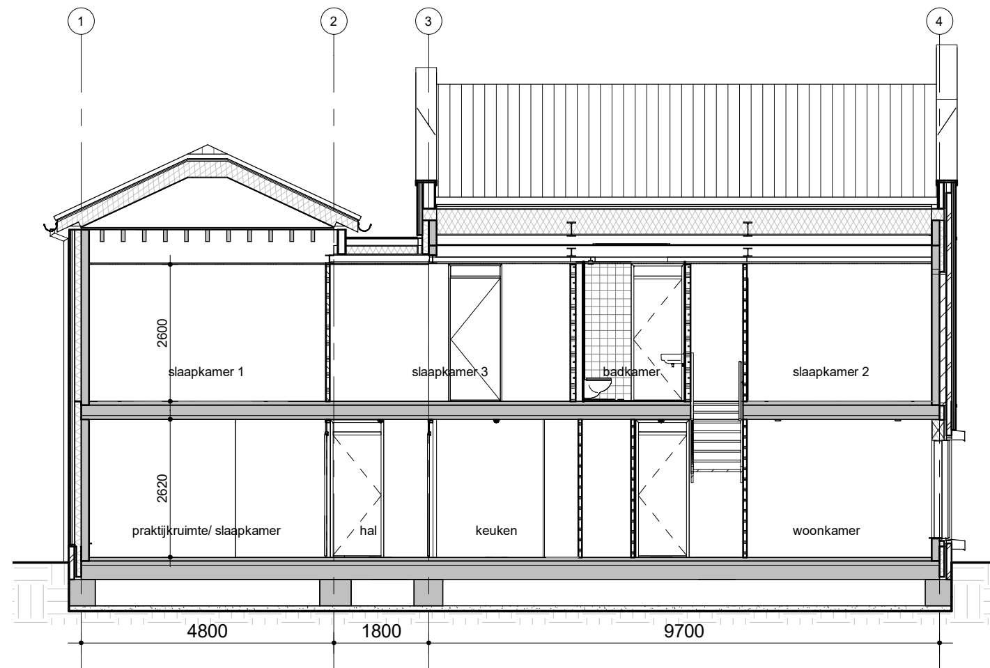
Doorsnede C
