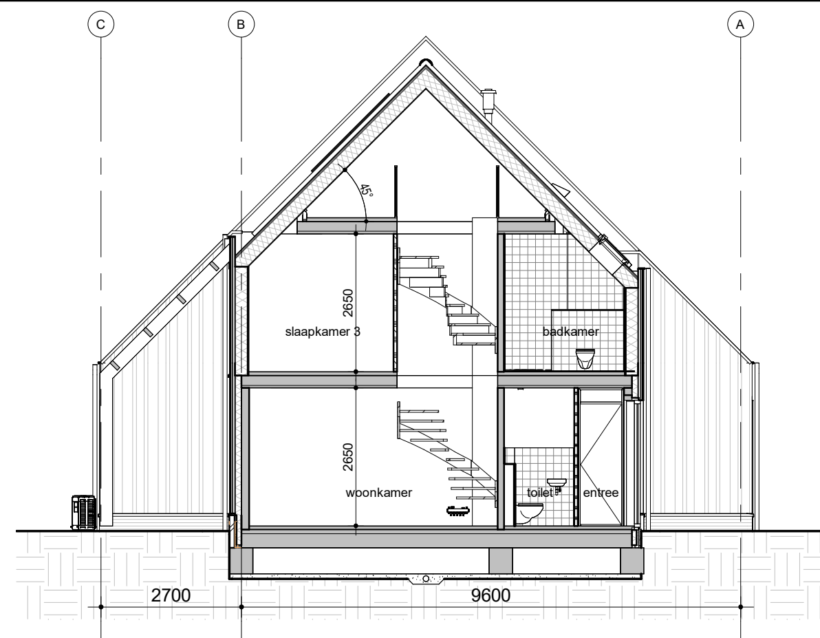
Doorsnede B
