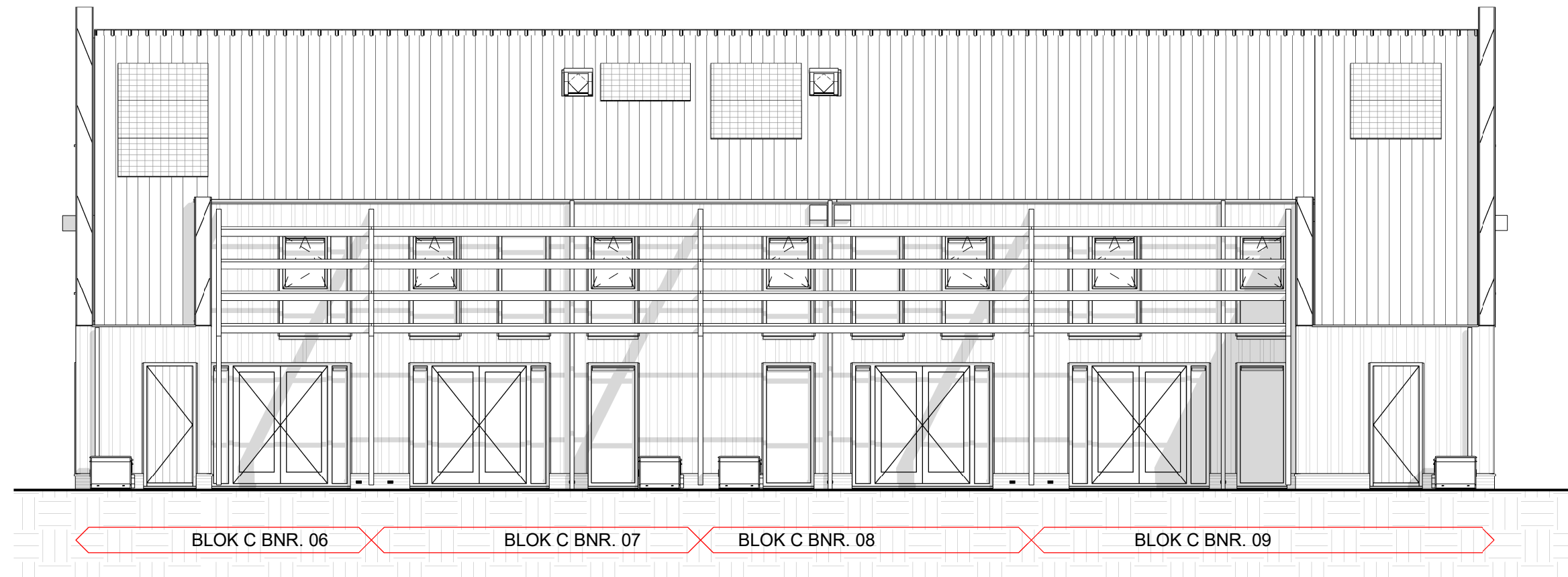
achtergevel
