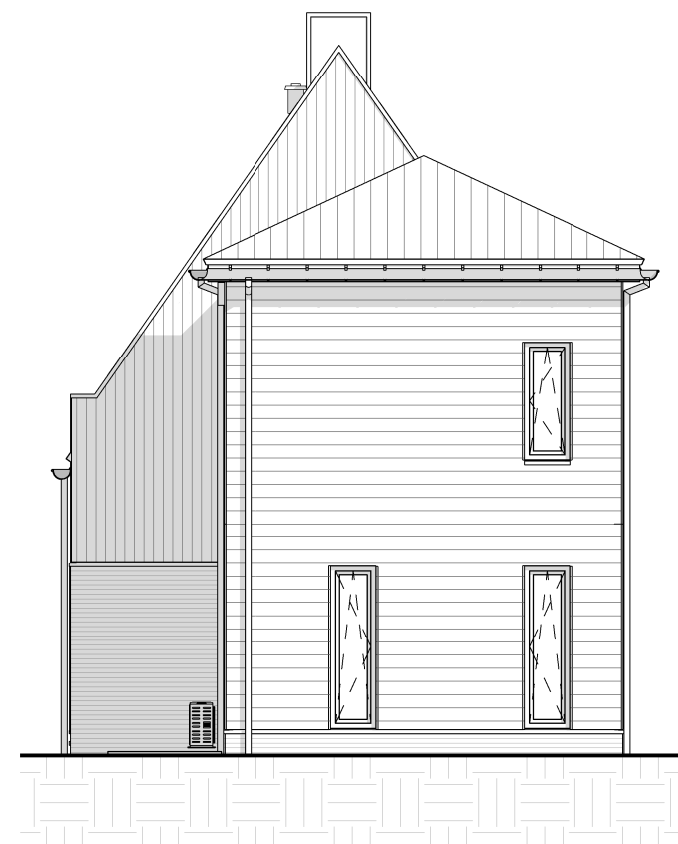
linkergevel
