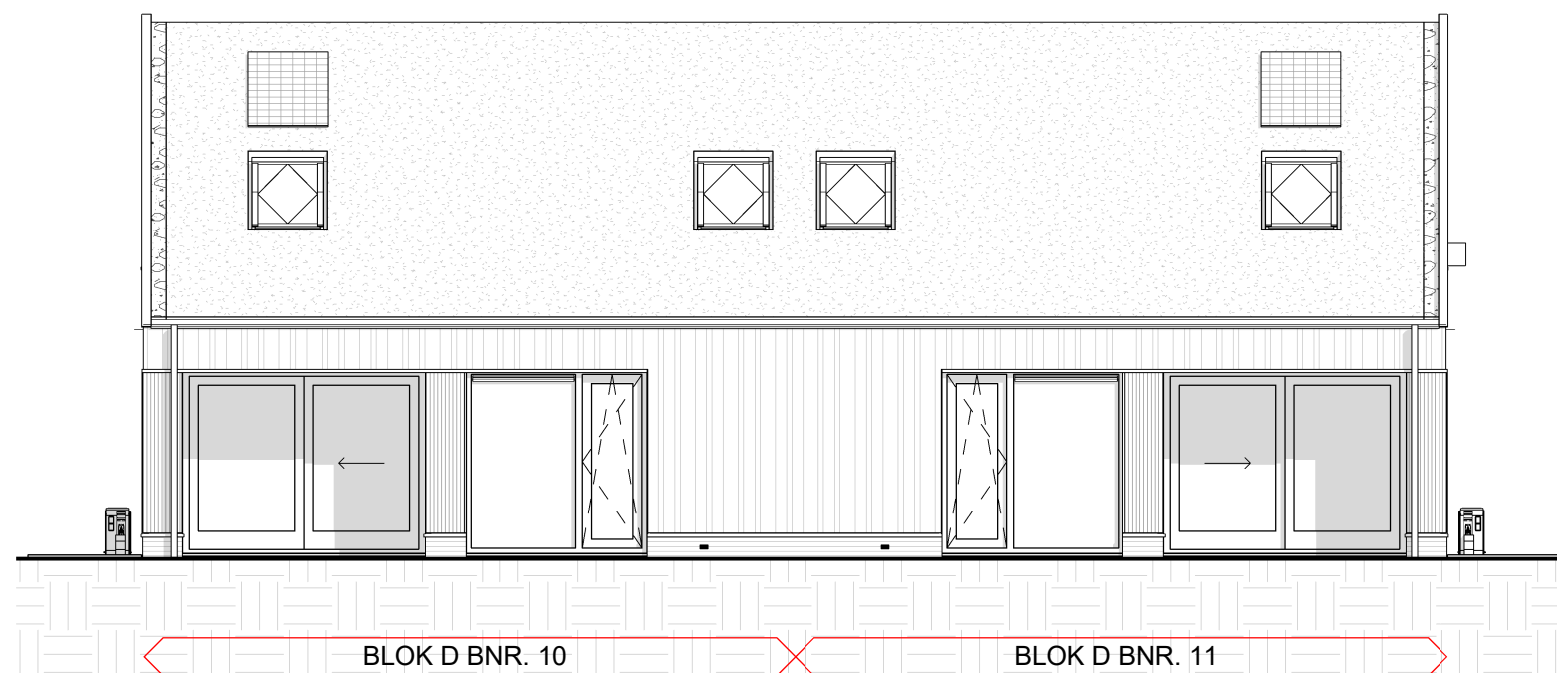
achtergevel
