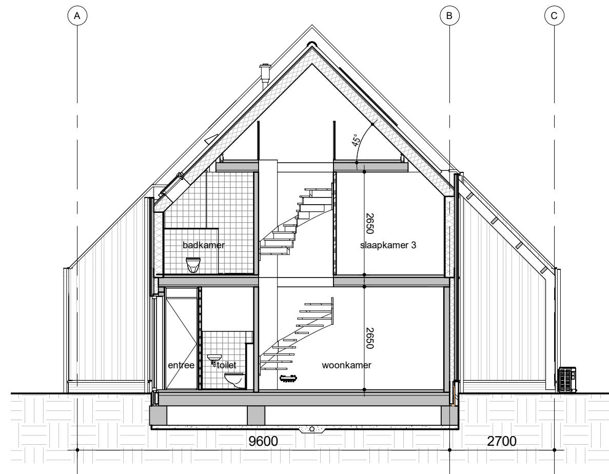
Doorsnede B
