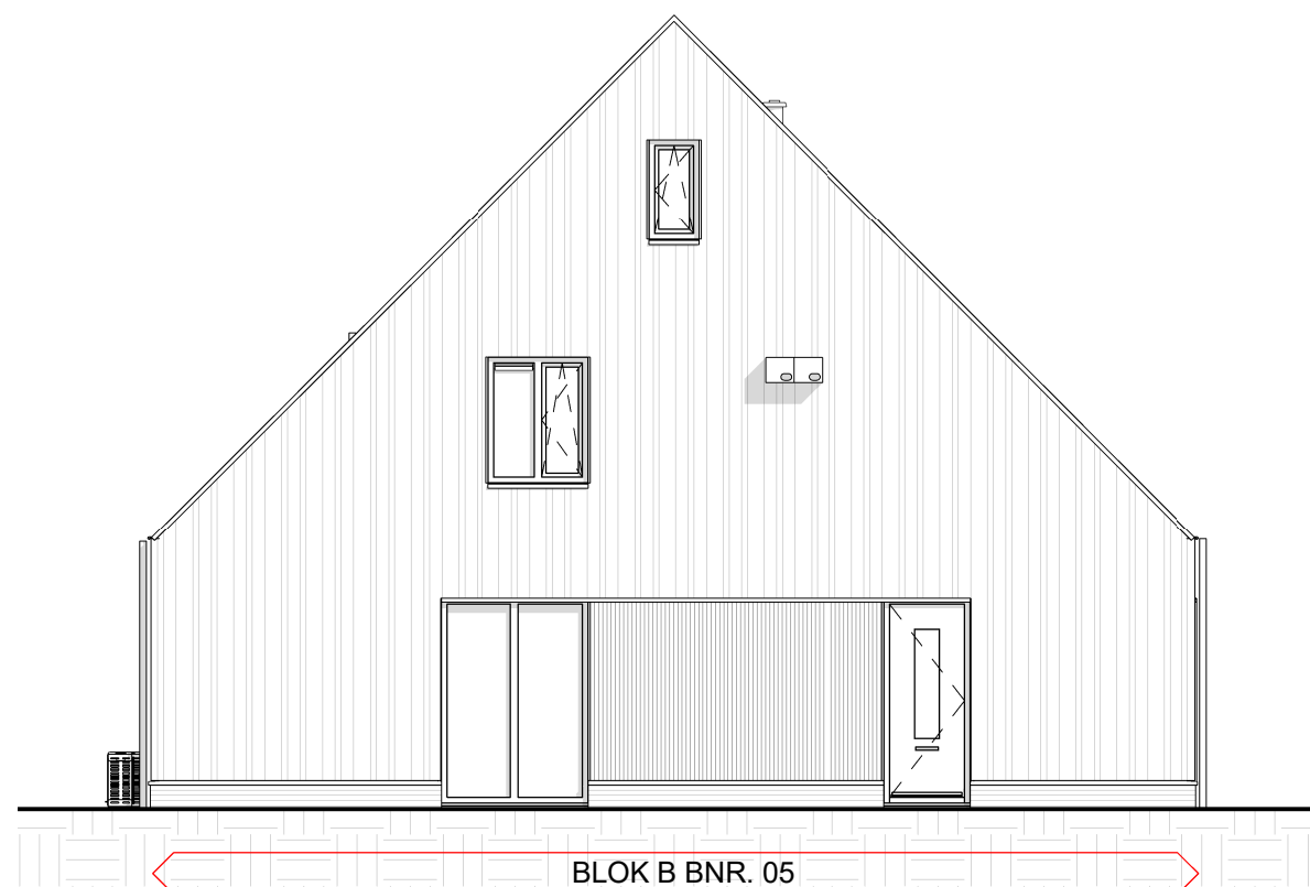
linkergevel
