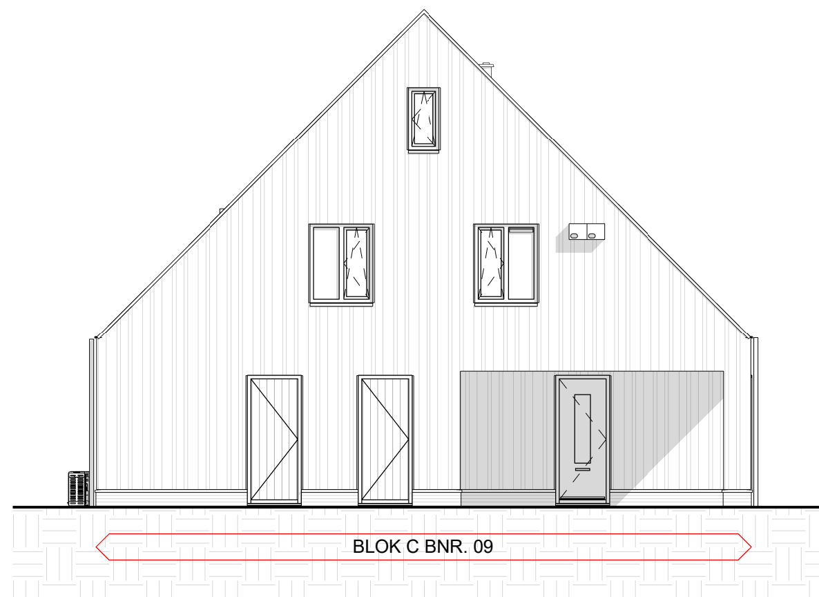
linkergevel
